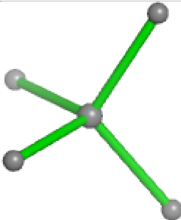
Bond angles
